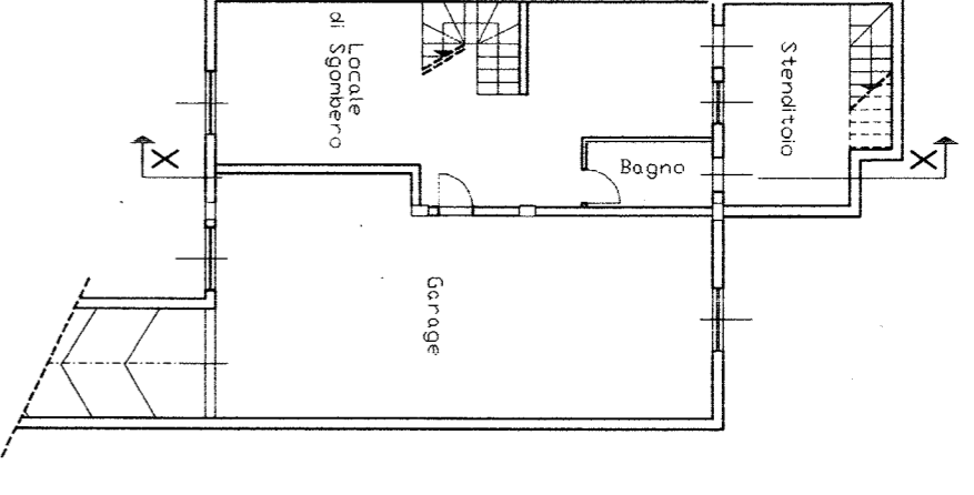
Piano Seminterrato scala 1:200
