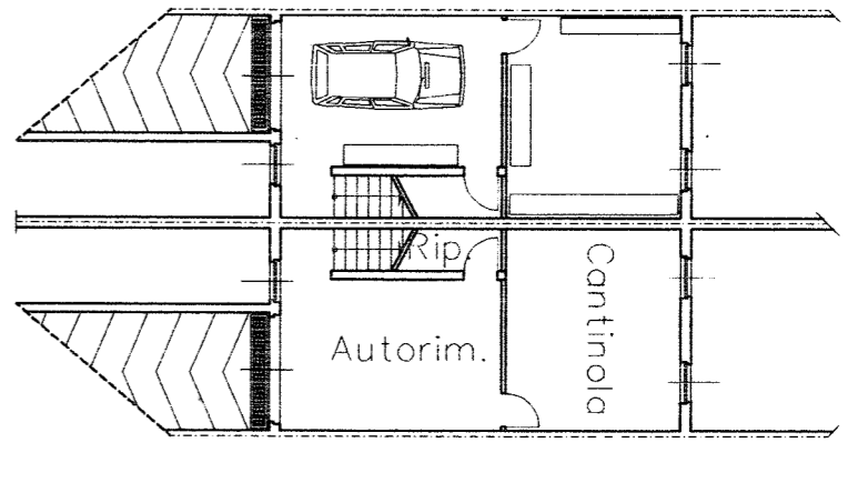
Piano Seminterrato scala 1:200
