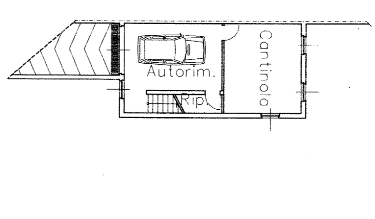
Piano Seminterrato scala 1:200
