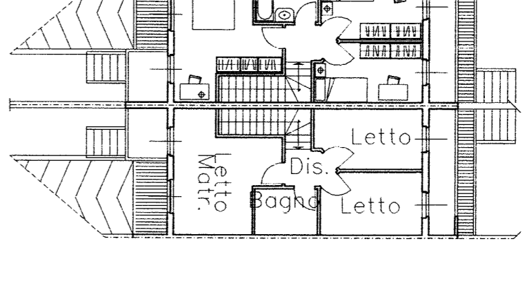
Piano Piano Primo scala 1:200
