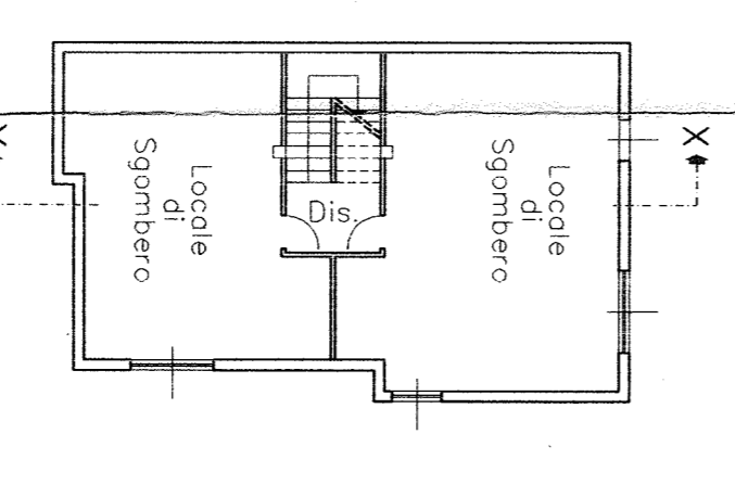
Piano Seminterrato scala 1:200
