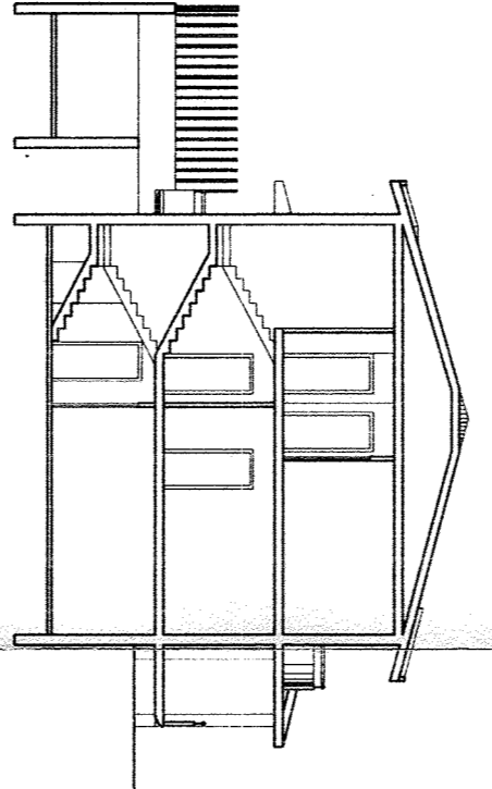
Sezione X - X scala 1:200
