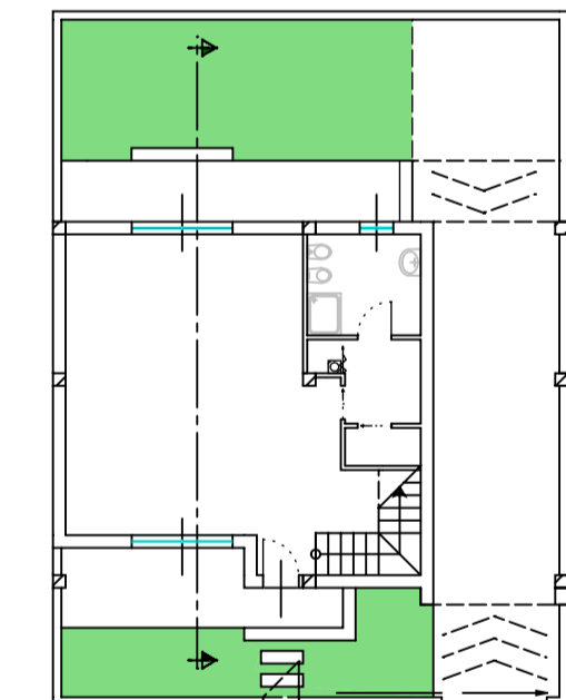
PIANO TERRA 1:200
