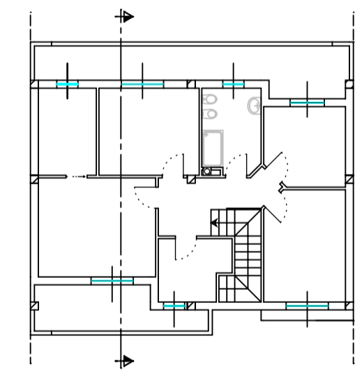
PIANO PRIMO 1:200
