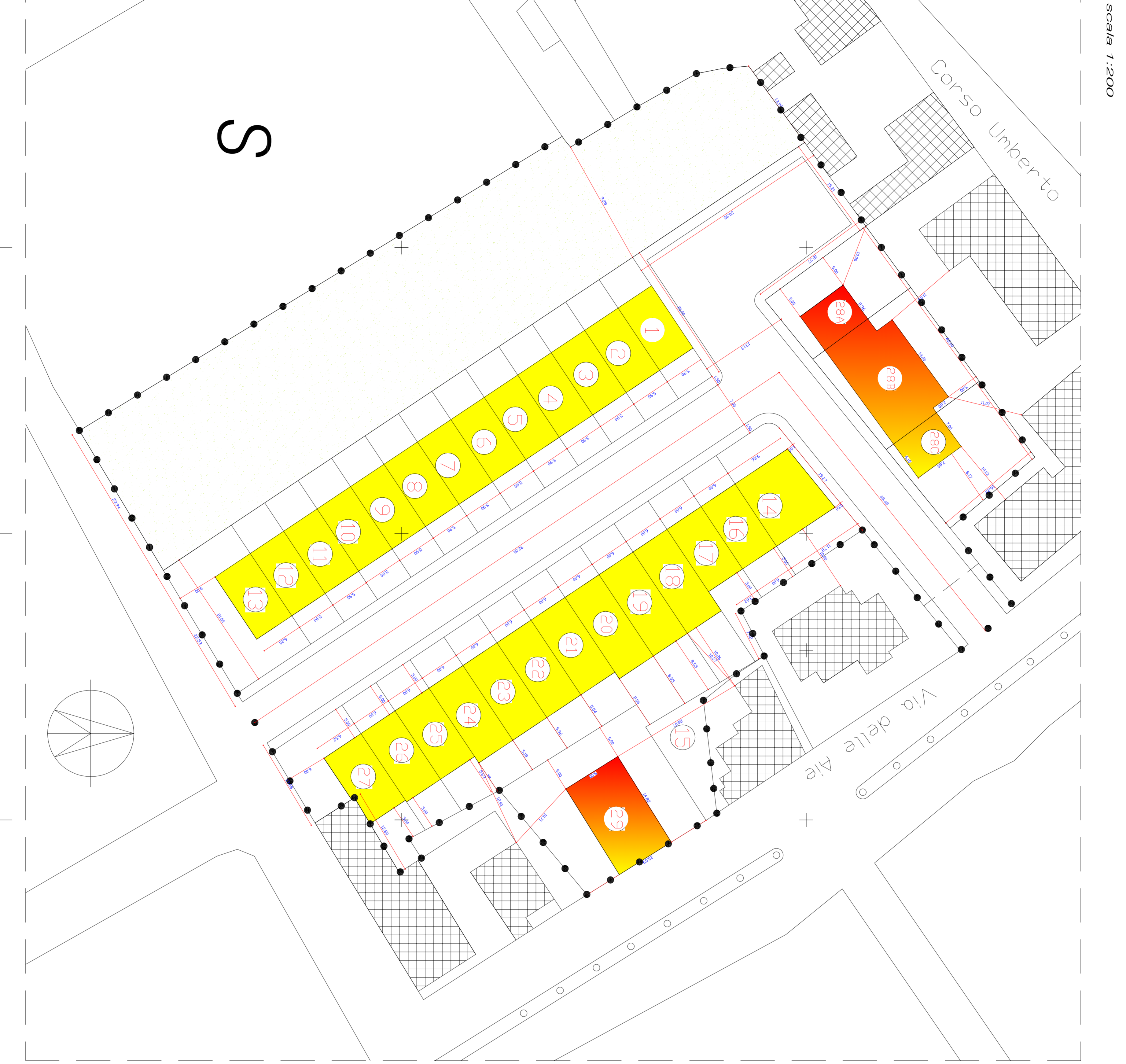
PIANTA PLANVOLUMETRICO APPROVATO
